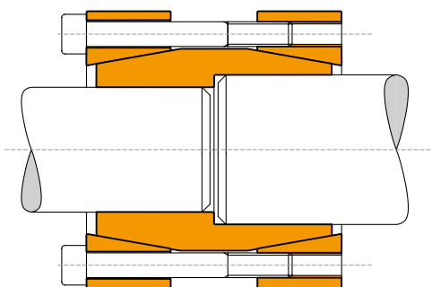
Doppeldurchmesserausführungen sind verfügbar
