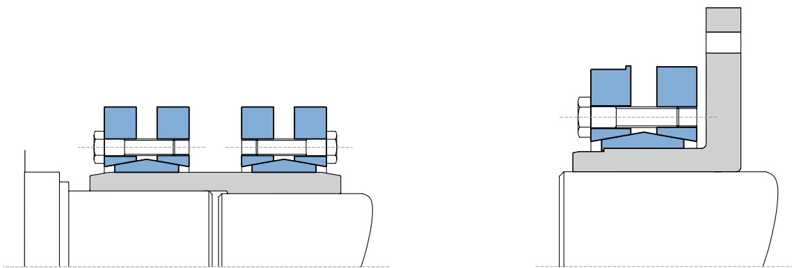
Verwendung von TLK603 als Kupplung zwischen Wellen mit verschiedenem Durchmesser
